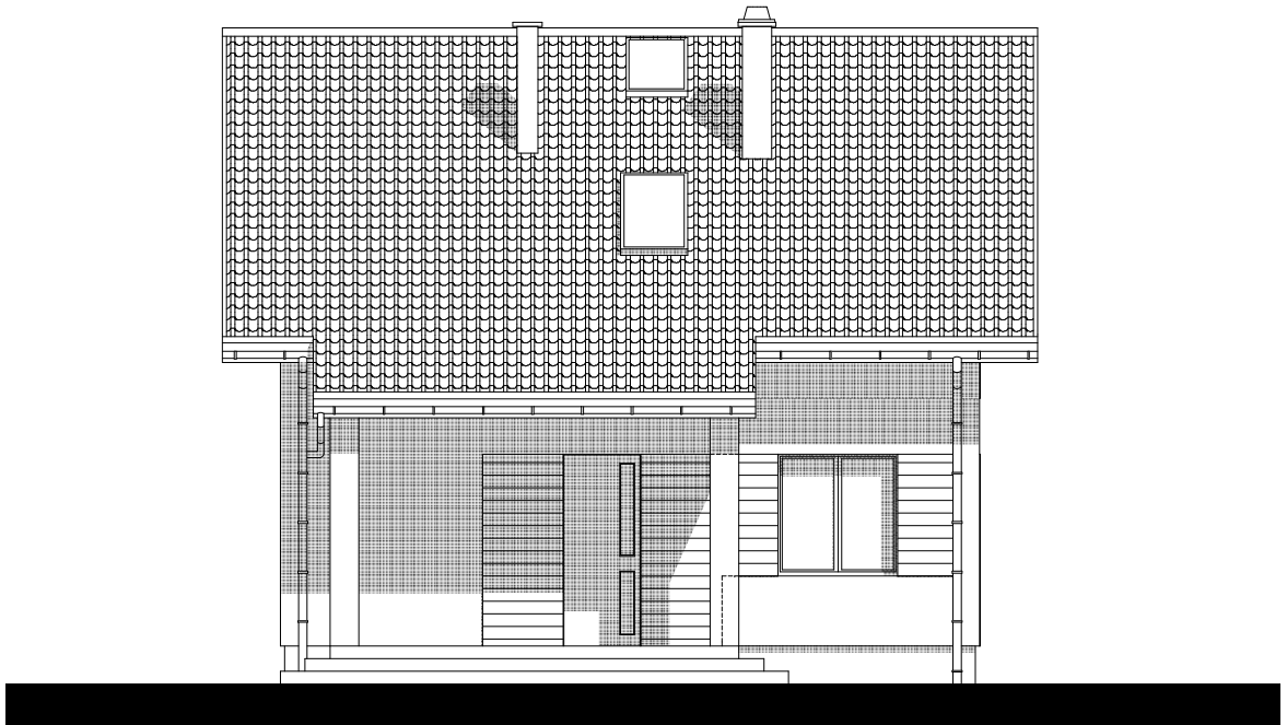
ELEWACJA...
