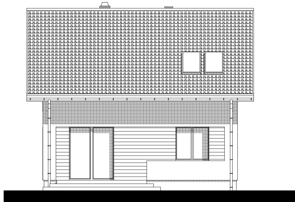
ELEWACJA...
